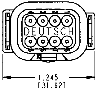
Deutsch Plug Connector P/N: DTM04-08PA
