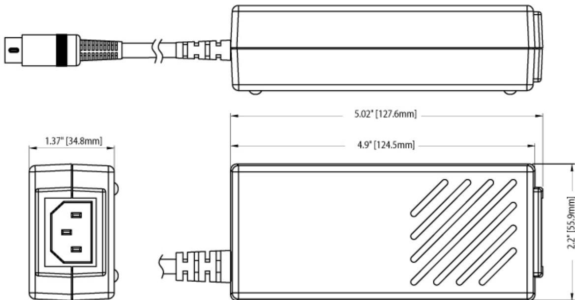
MWA065-DWG
